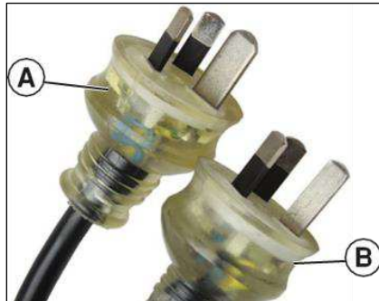
A - 15 Ampere
