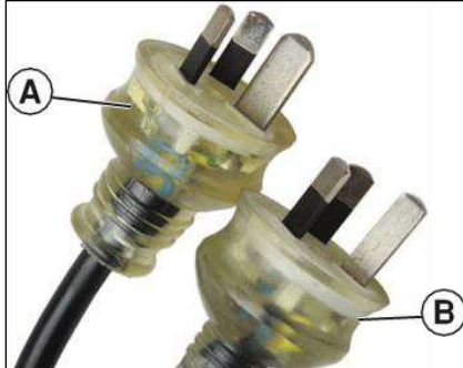
A - 15 Ampere B - 10 Ampere
